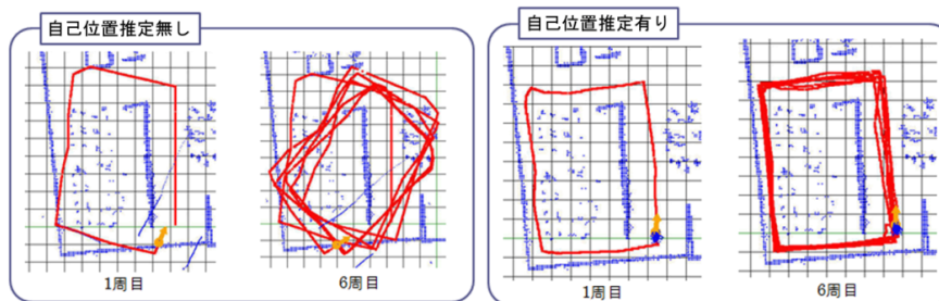
図 6 位置推定あり・なしの場合のそれぞれの移動軌跡
