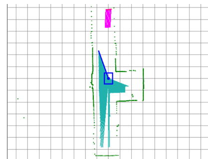
図 2 レンジセンサによる障害物情報の取得
