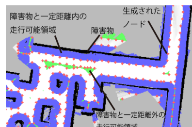
図 7 地図上の障害物とその境界線
