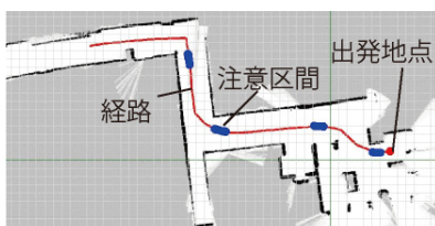
図 12 使用した経路とその注意区間
