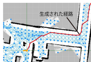
図 8 地図に付与されたグラフ構造データと生成された経路
