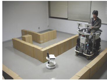
図 17 注意区間で停止した SUV とそのときの AT のコンソール画面
