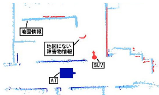
図 14 SUVによるATのセンシング領域の拡張
