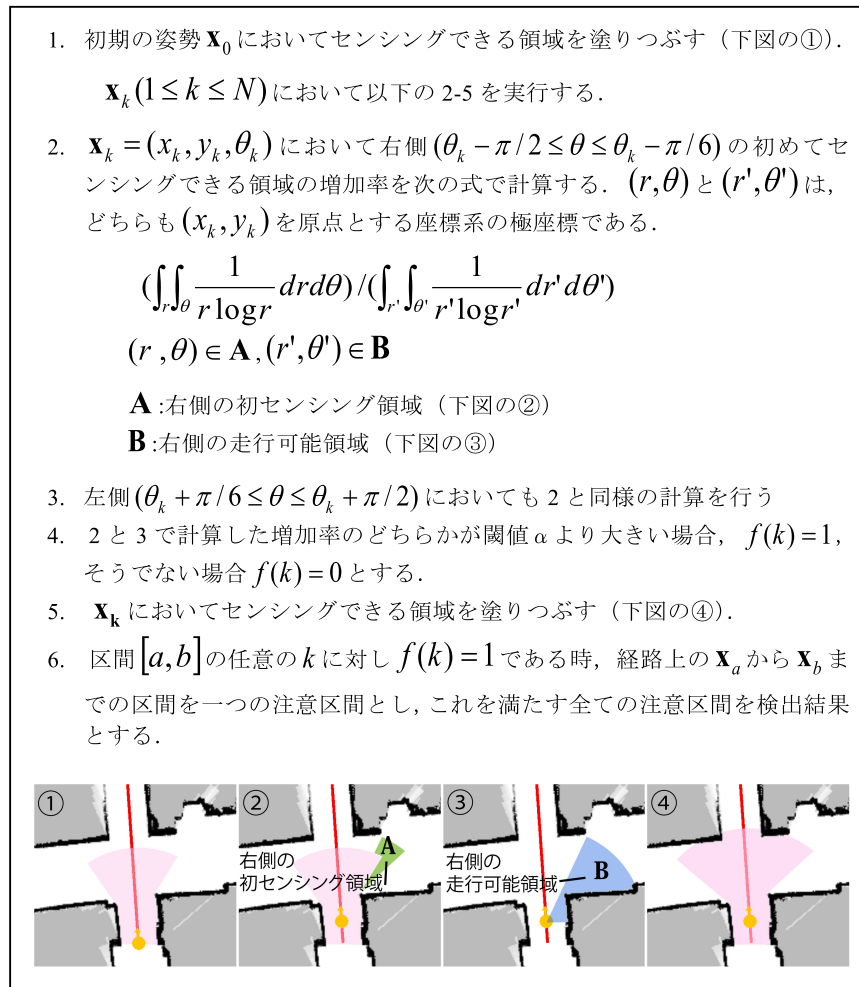
図 10 注意区間の検出アルゴリズム
